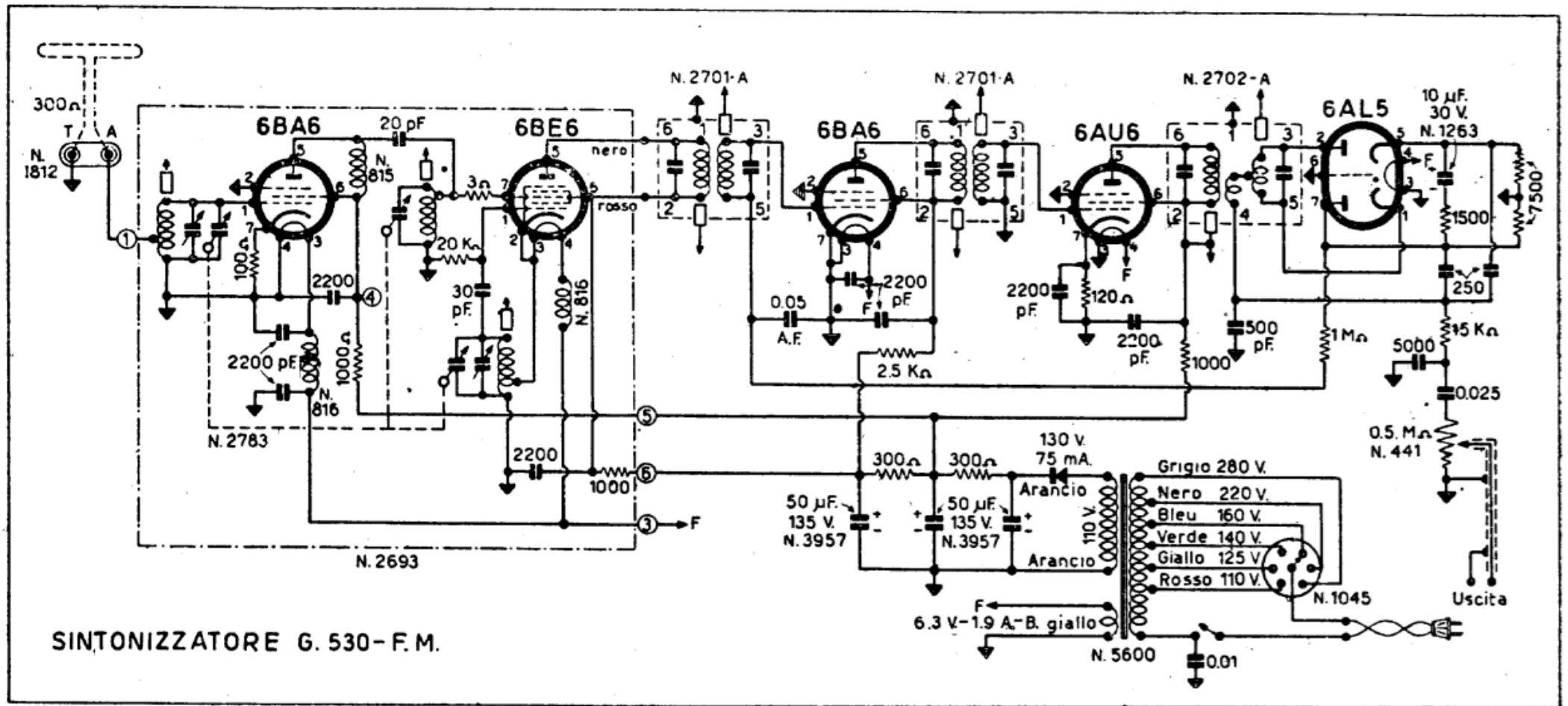
Fig. 4 - Lo schema elettrico.
